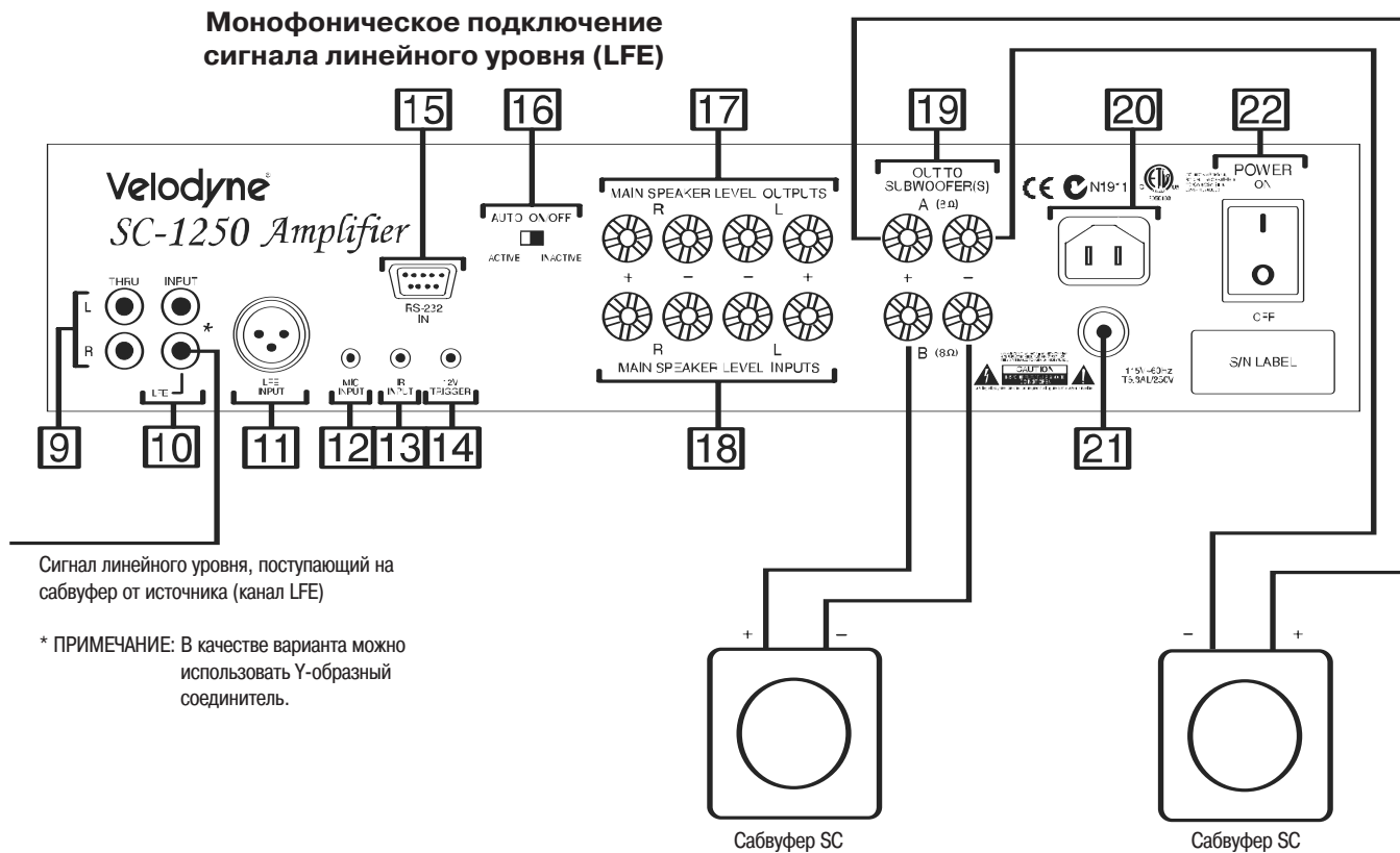
Рис 3А: Монофоническое подключение (канал низкочастотных эффектов LFE) сигнала линейного уровня.
